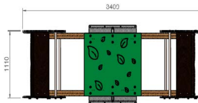
PLANTA Cotas en mm
