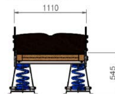
PERFIL Cotas en mm
