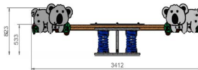
ALZADO Cotas en mm
