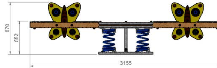
ALZADO Cotas en mm
